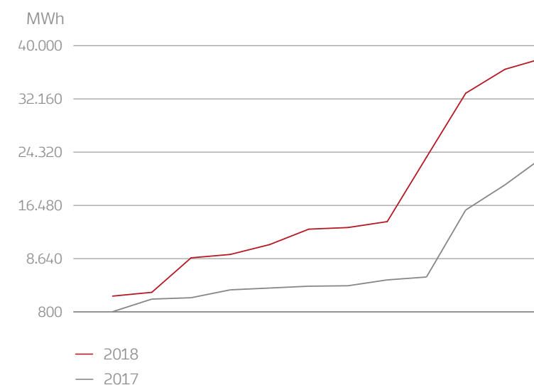
Total realiseret vindregulering i MWh for 2017 og 2018
